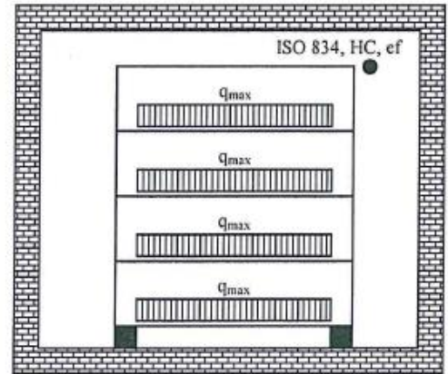
Fig. 2: SEZIONE VERTICALE
